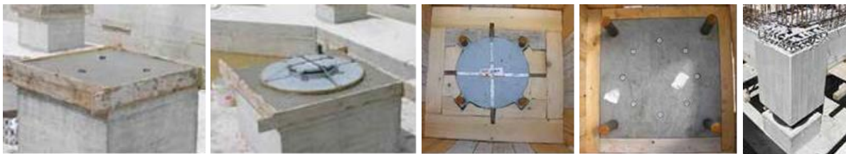
Immagine 27: Procedura d'installazione di isolatore friction pendulum su una nuova costruzione.
