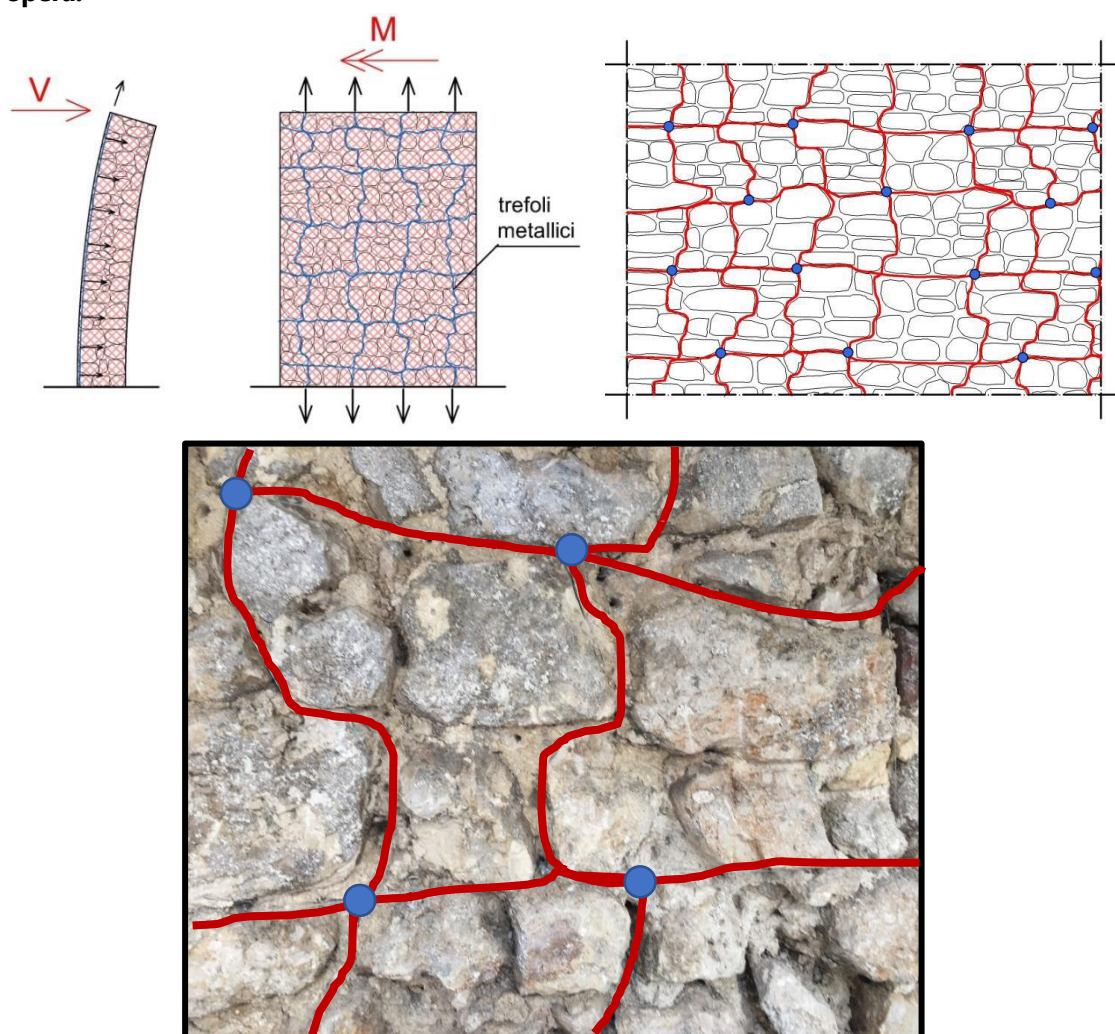
Immagine 18: Sistema ANCHORSTEEL NET per muratura irregolare.
