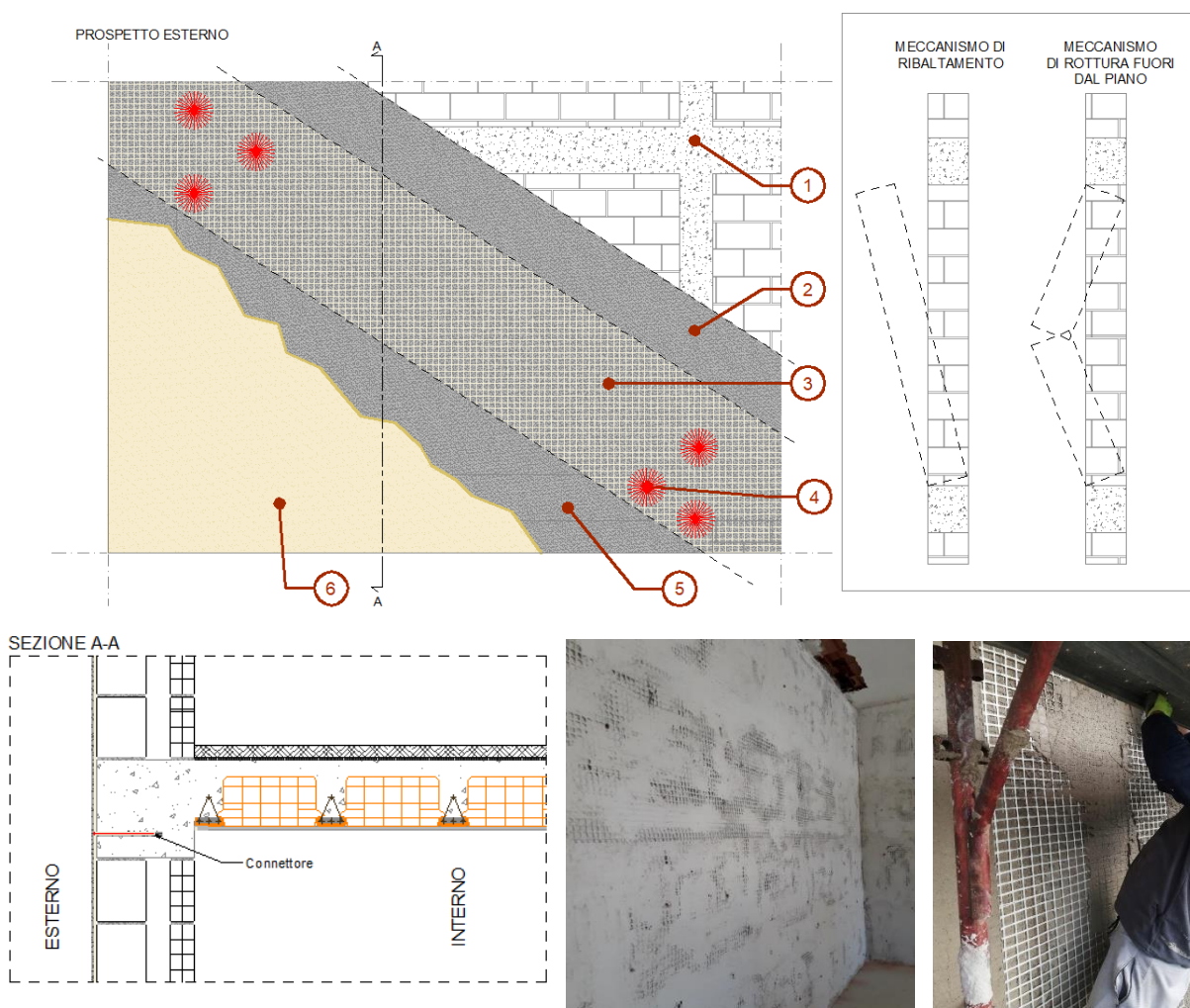
Immagine 10: Sistema antiribalta diffuso.
